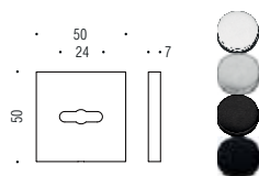
PB23/06 MOSTRINA QUADRATA PER DOPPIA MAPPA UNIVERSALE SQUARE ESCUTCHEON FOR UNIVERSAL DOUBLE BITTED KEY
