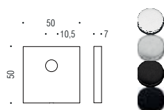
PB23/05 MOSTRINA QUADRATA PER CILINDRO CON POMOLO SQUARE BACKPLATE FOR CYLINDER WITH KNOB
