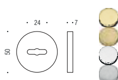
PB13/06 MOSTRINA TONDA PER DOPPIA MAPPA UNIVERSALE ROUND ESCUTCHEON FOR UNIVERSAL DOUBLE BITTED KEY
