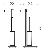
B9108 Piantana con doppio porta rotolo e porta scopino Floor standing column with double paper holder and brush holder
