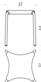
B9955 SIT Sgabello. Seduta: in ABS bianco Struttura: in alluminio verniciato con polverepossidica grigia SIT Seat. Seat: white ABS. Frame: grey epoxy powder coated aluminium
