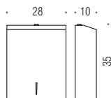
B9960N Distributore di salviette di carta con serratura di sicurezza - acciaio inox. Capienza max fogli carta piegata a «C», 400 salviette, misura 220x95mm Stainless steel paper tissue dispenser with safety lock. Maximum capacity of "C" folded paper sheets, 400 tissues, 220x95mm size
