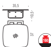
B9645 Sedile doccia ribaltabile con finitura fotoincisa antiscivolo, completo di staffa a muro Tilt-up shower seat with antislip finish, complete with wall bracket
