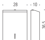
B9960N Distributore di salviette di carta con serratura di sicurezza - acciaio inox. Capienza max fogli carta piegata a «C», 450 salviette, misura 270x96mm Stainless steel paper tissue dispenser with safety lock. Maximum capacity of "C" folded paper sheets, 450 tissues, 270x96mm size
